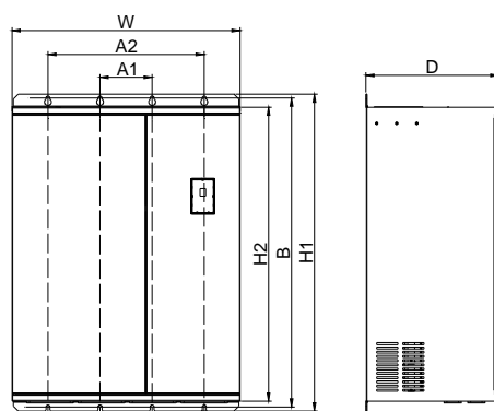
AE300 系列 280-1400KW (无底座)
