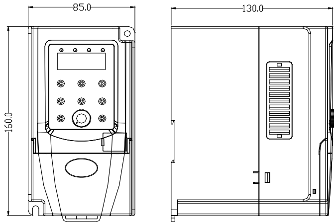
AE300X 系列 0.75-4KW 尺寸图(单管机器)
