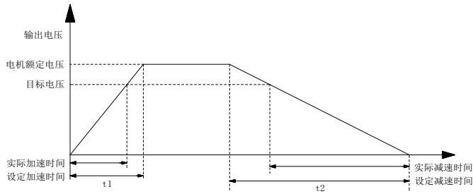
V/F 分离示意图
