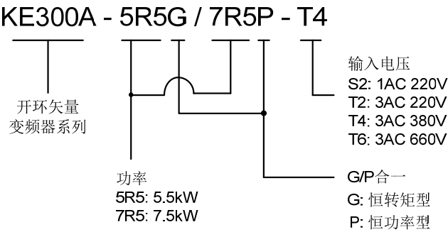
图 2-1 型号说明
