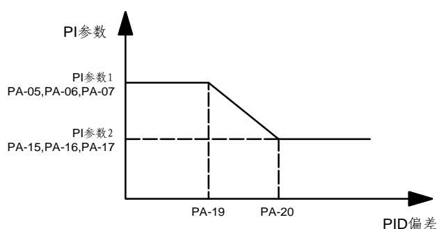
图 6-25 PID 参数切换
