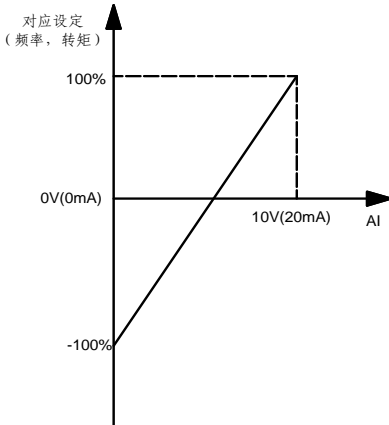
图 6-9 模拟给定与设定量的对应关系
