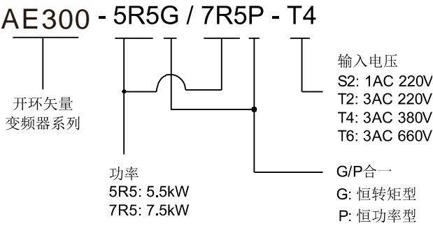
图 2-2 型号说明
