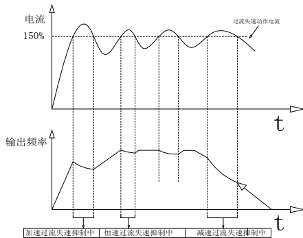
过流失速动作示意图
