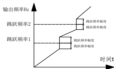
图 6-17 加减速过程中跳跃频率有效示意图
