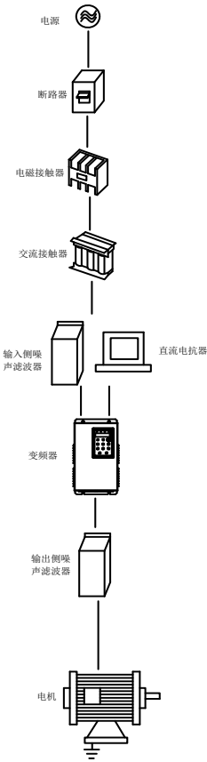
图 3-2 KE300A&AE300 变频器与外围机器的连接示例
