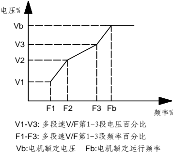
图 6-4 多点 V/F 曲线设定示意图
