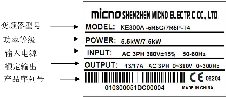
图 2-3 铭牌说明
