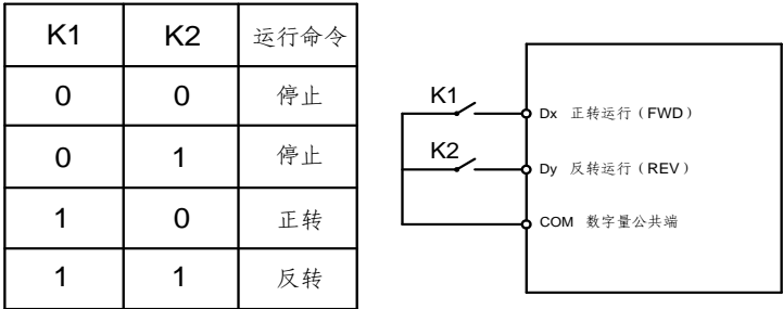
图 6-6 两线式模式 2
