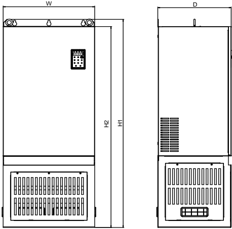
132~250kW 非标机（有底座）
