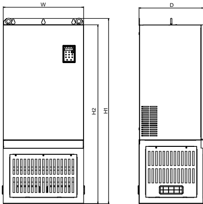
160~200kW (有底座, 需非标定制)
