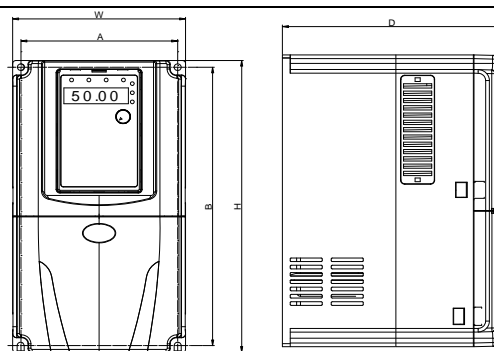
AE300 系列 0.75~11kW 尺寸图
