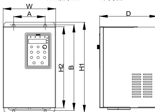
15~45kW 尺寸图
