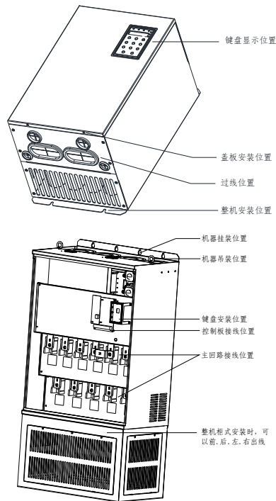
图 2-3 变频器各部件说明
