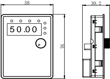
单相/三相 220V 0.4-1.5KW 变频器用 58*76mm 键盘尺寸(KE300X 系列)
