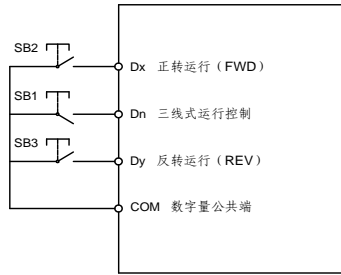
图 6-7 三线式控制模式 1
