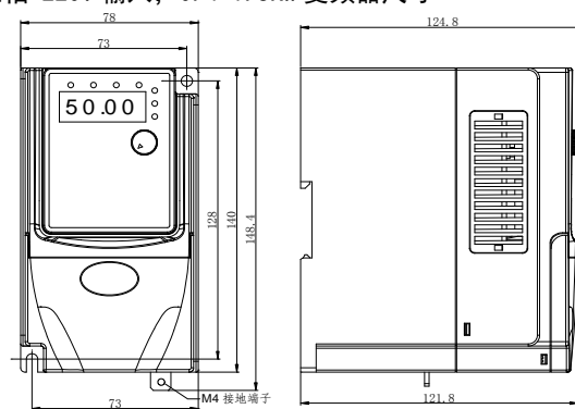
KE300X 系列 0.4~1.5KW
