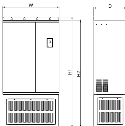
AE300 系列 280-1400KW (带底座)
