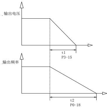
V/F 分离输出电压/频率独立减至 0
