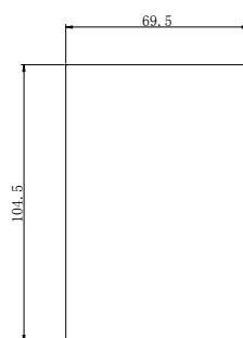
65*100mm 键盘托架开孔尺寸
