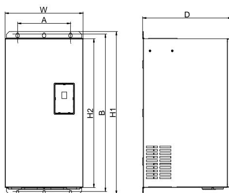
55~250kW 尺寸图 (含 132~250kW 的标准机)
