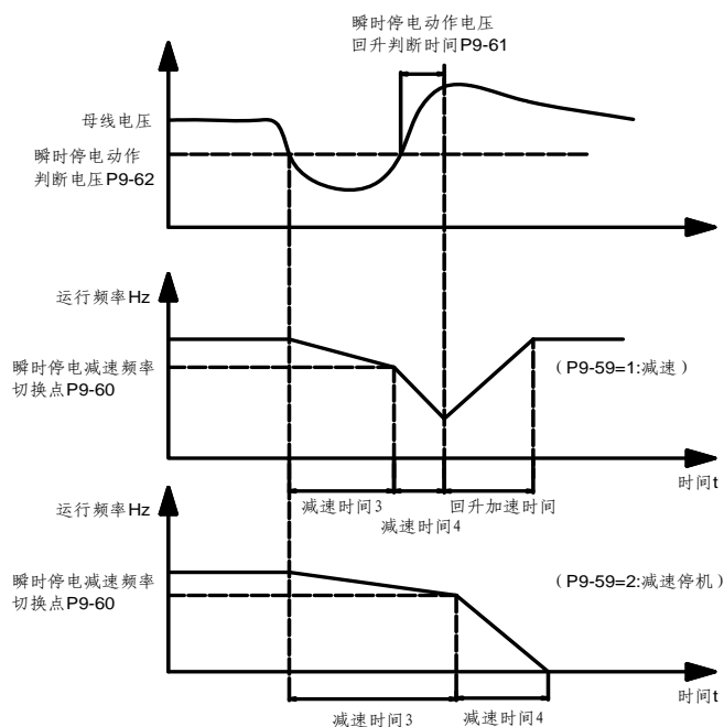
图 6-23 瞬时停电动作示意图
