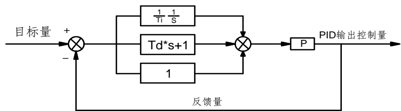
图 6-24 过程 PID 控制原理框图
