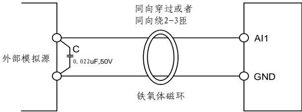
图 3-16 模拟量输入端子处理接线图
