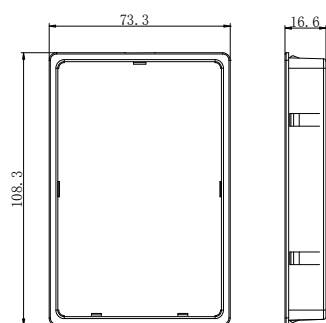
65*100mm 键盘托架尺寸
