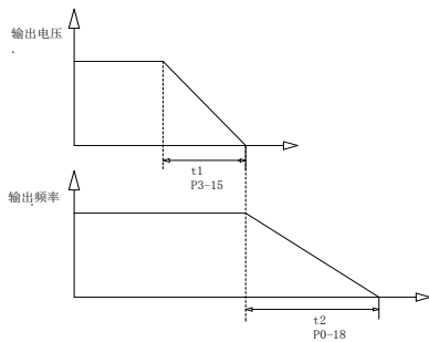
V/F 分离频率 / 电压先后下降示意图
