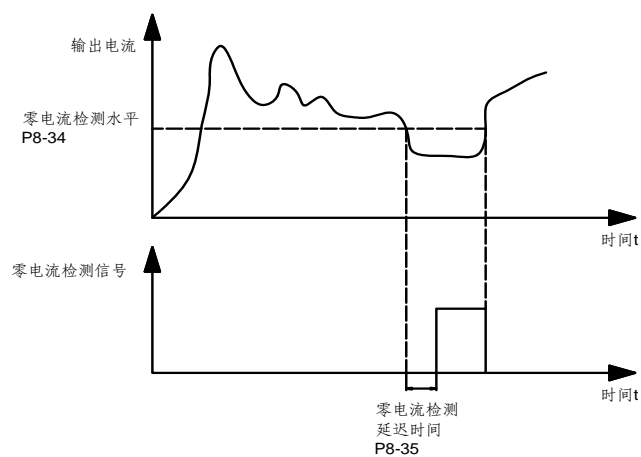
图 6-20 零电流检测示意图
