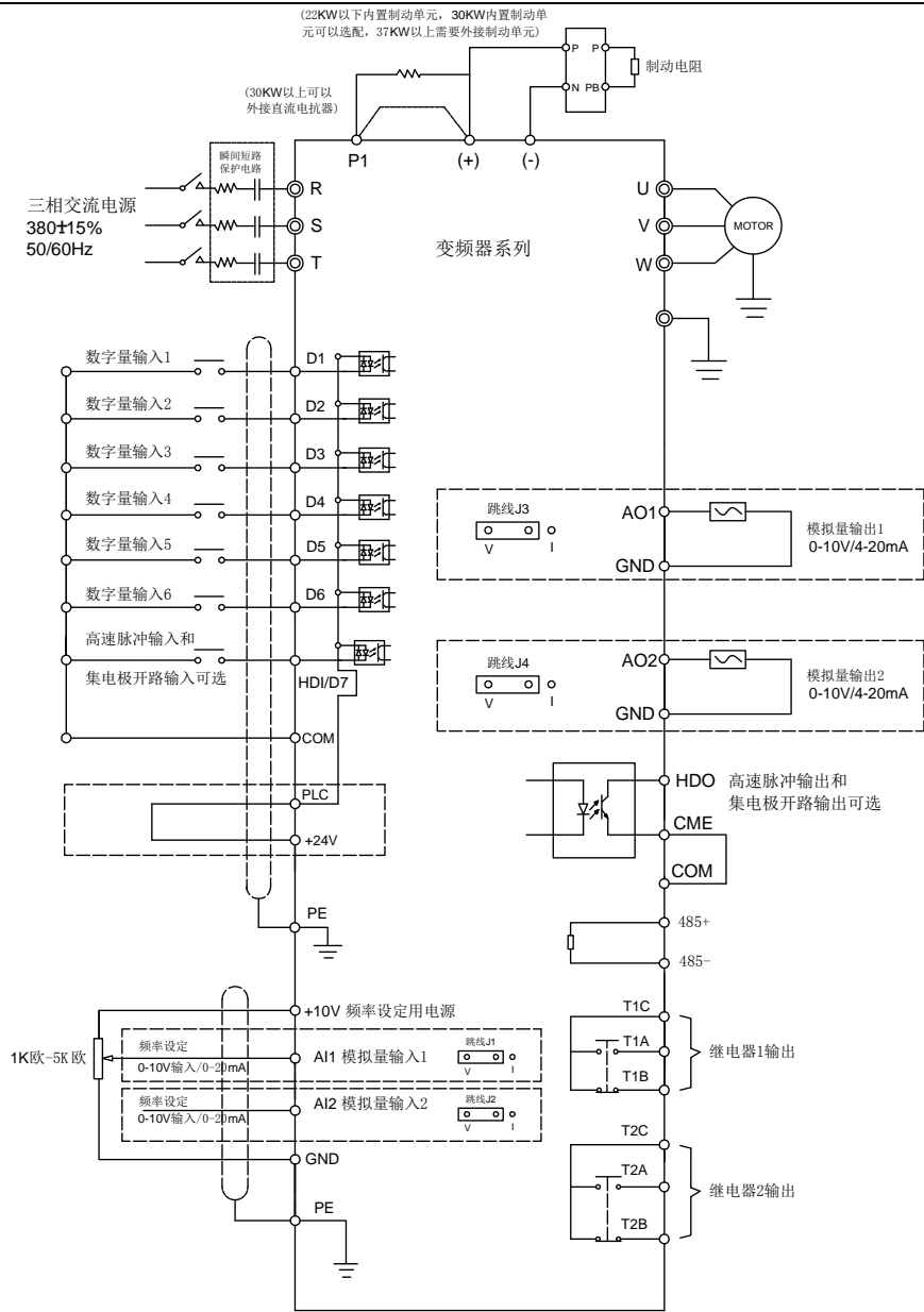
图 3-4 其它功率变频器接线图
