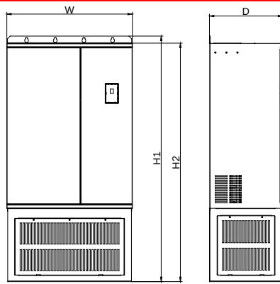
280-1600KW (690V) 有底座
