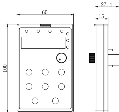
65*100mm外引键盘尺寸
