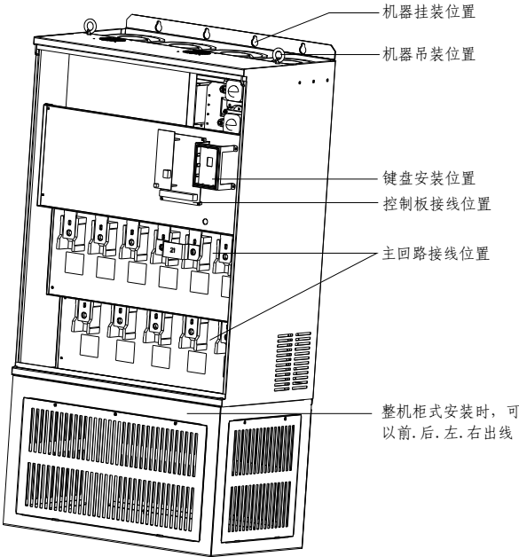
图 2-3 驱动器各部件说明
