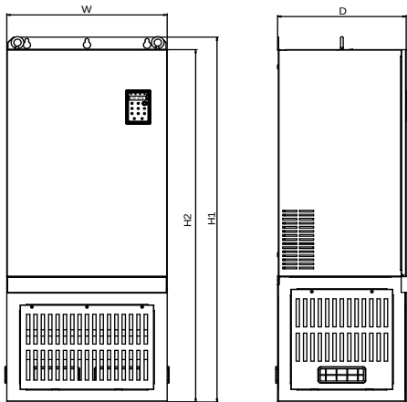
132-250kW 非标机（有底座）
