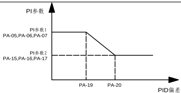
图 6-25 PID 参数切换
