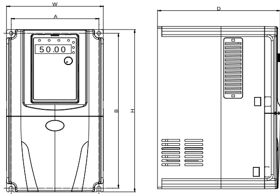
0.75-11KW 尺寸图
