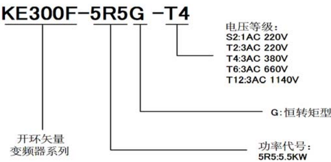
图 2-2-1 型号说明
