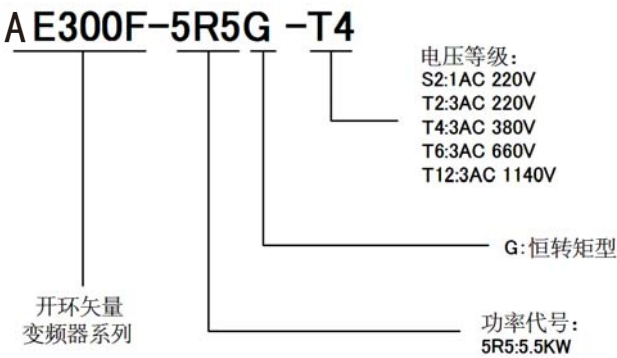
图 2-2-2 型号说明
