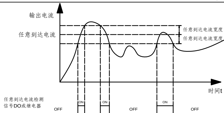
图 6-22 任意到达电流检测示意图
