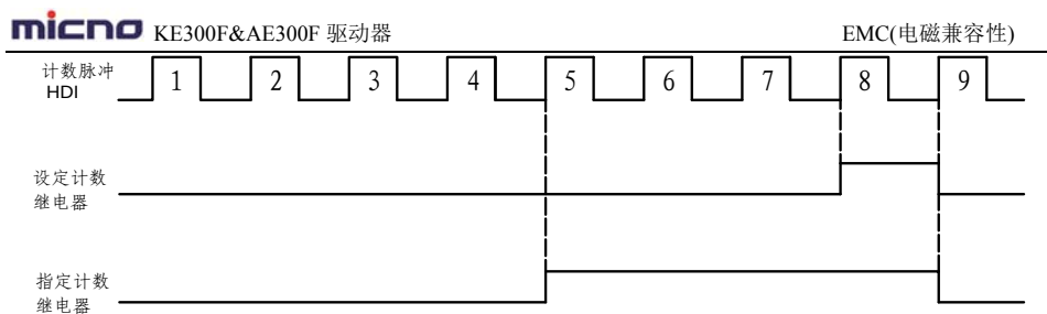
图 6-28 设定计数值给定和指定计数值给定示意图
