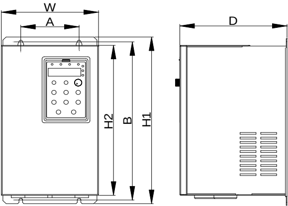
15-45KW 尺寸图
