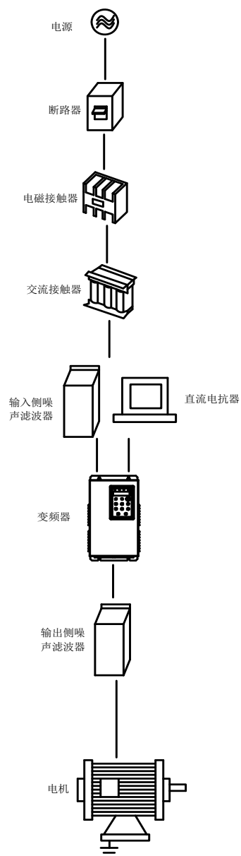
图 3-2 KE300F&AE300F 驱动器与外围机器的连接示例
