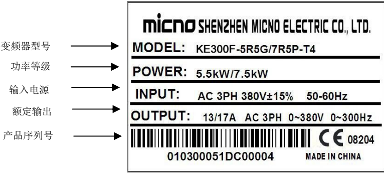
图 2-3-1 铭牌说明
