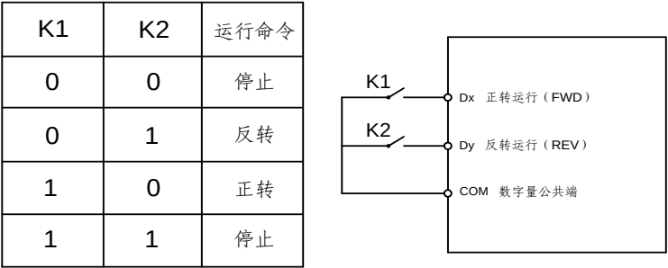
图 6-5 两线式模式 1
