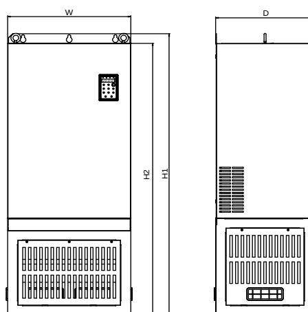
90~200kW 非标机 (有底座)
