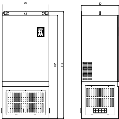
160~200kW（有底座，需非标定制）
