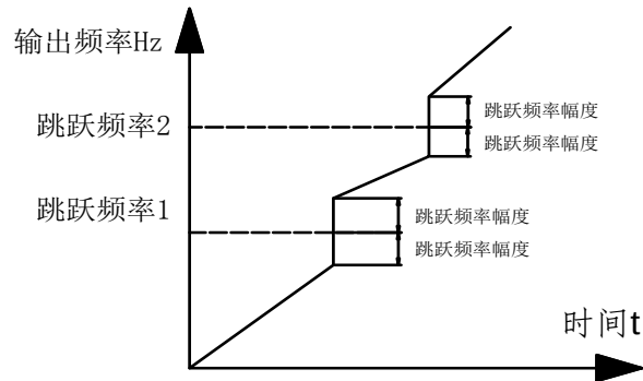
图 6-17 加减速过程中跳跃频率有效示意图
