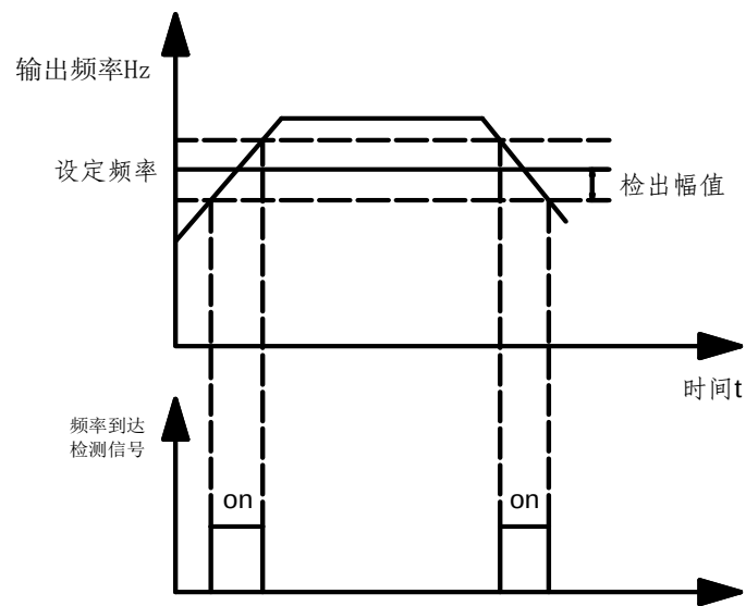
图 6-16 频率到达检出幅值示意图
