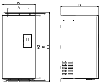
55-250KW 尺寸图（含 132~250kW 的标准机）
